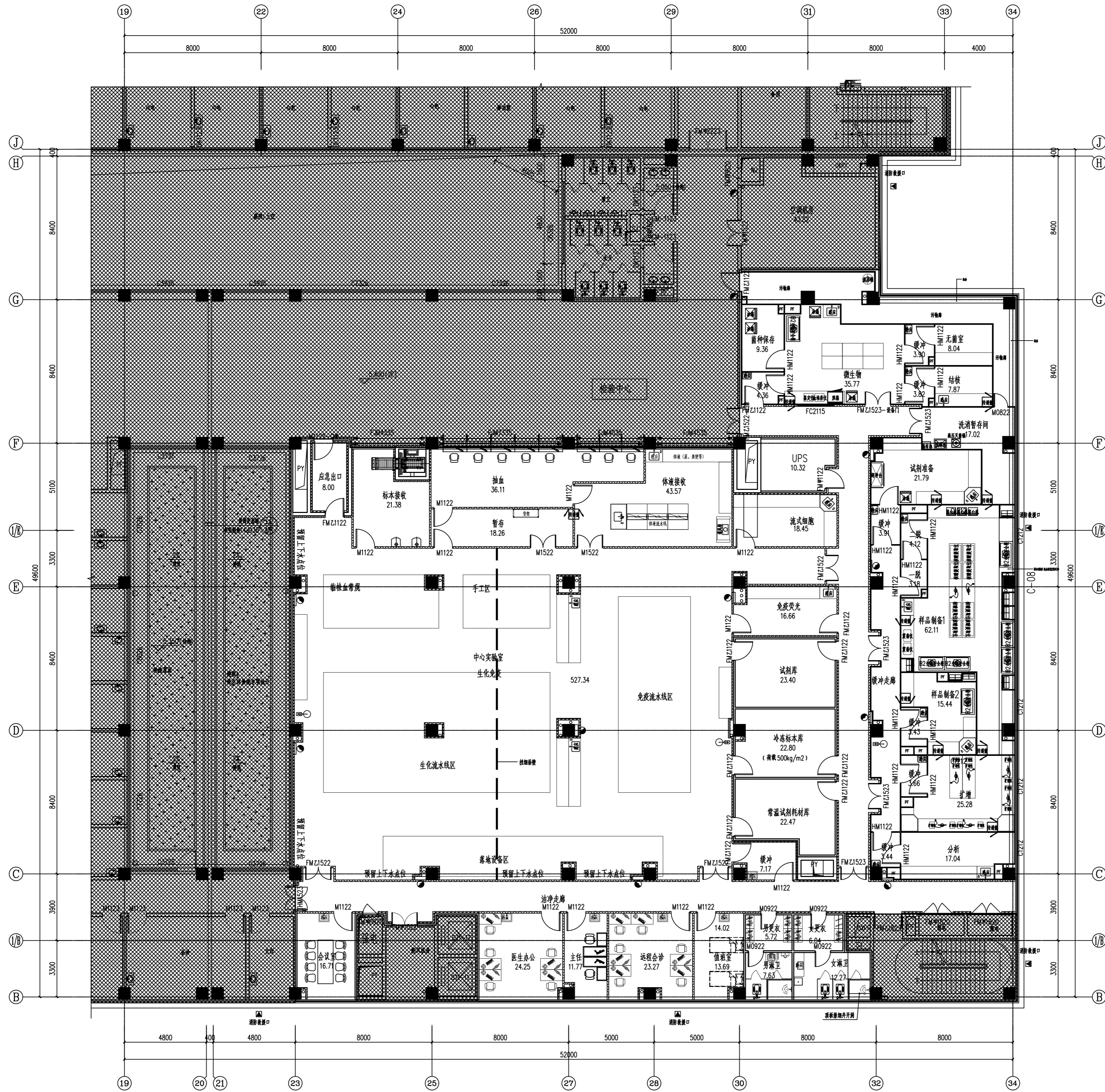
二层检验中心平面布置图 1:50
